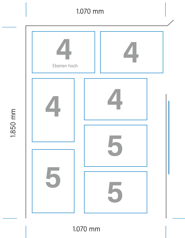
Heckeinsicht maximale Grundbeladung mit E2-Kisten
